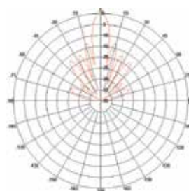
H-Plane Pattern
